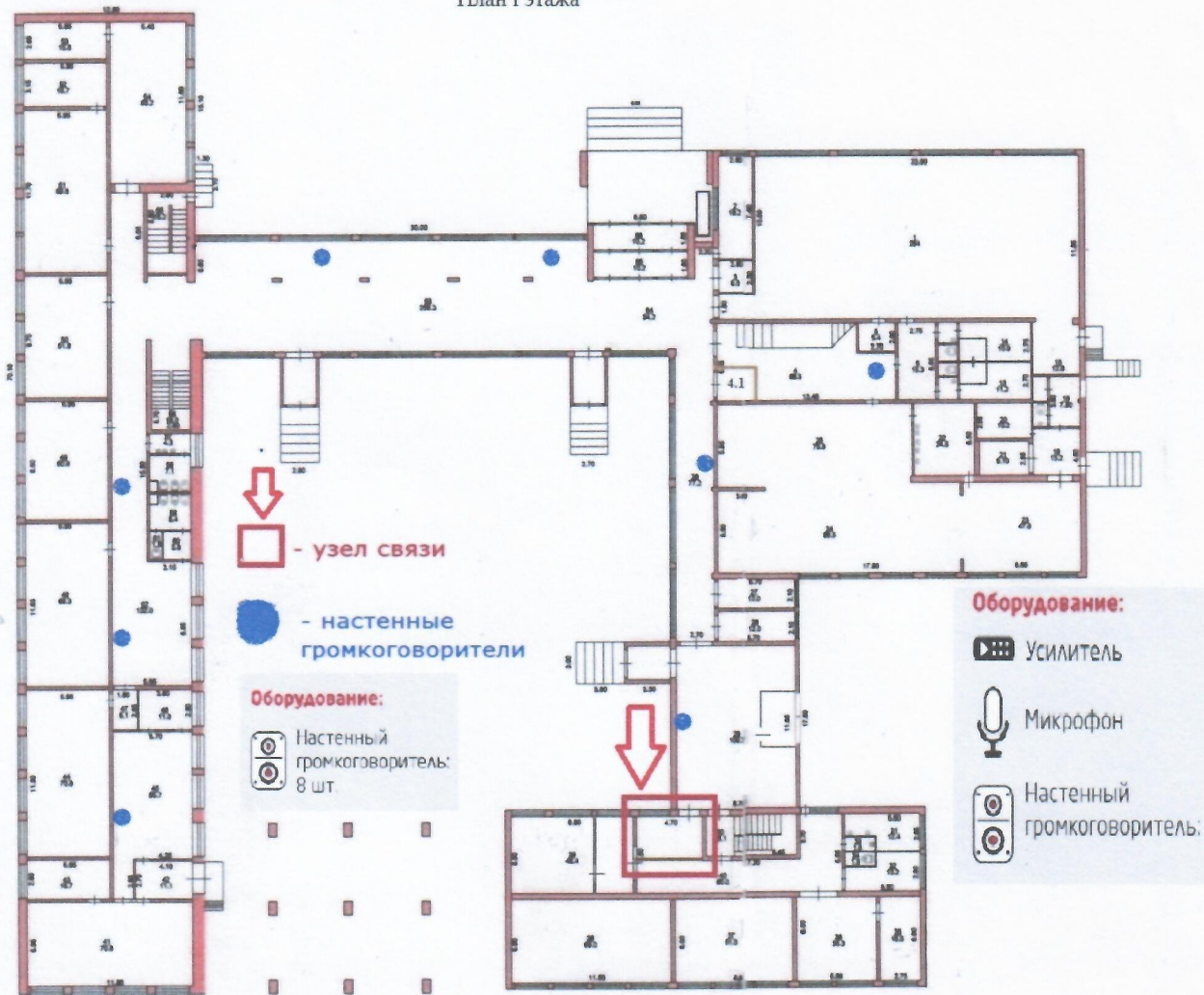
План I этажа
